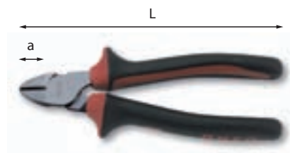
185 B UNI DIN ISO 5749
