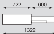
Cassetto con guida telescopica ad estrazione totale portata kg 120
